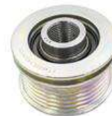
FT45705 POULIE ROUE LIBRE, ALTERNATEUR ROUE LIBRE 1.5/2.0/2.2 HDI
